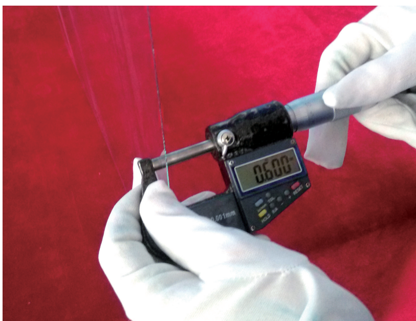
工作人员测量刚下线的超白超薄玻璃厚度
