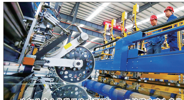
汝阳县产业集聚区洛玻集团Low-E镀膜玻璃生产线
