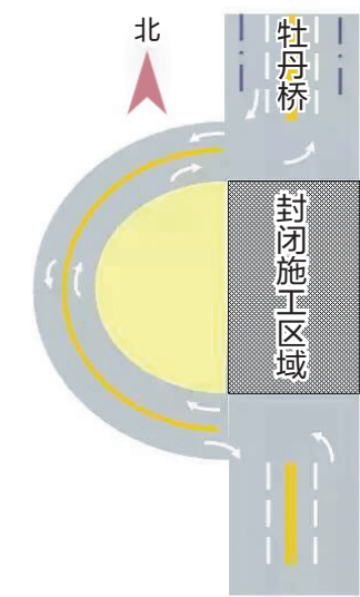
滨河南路下穿牡丹桥工程车辆绕行示意图
