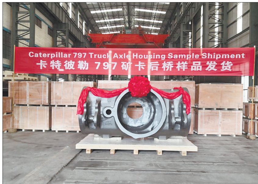
铸件全貌 记者 赵志伟 摄
