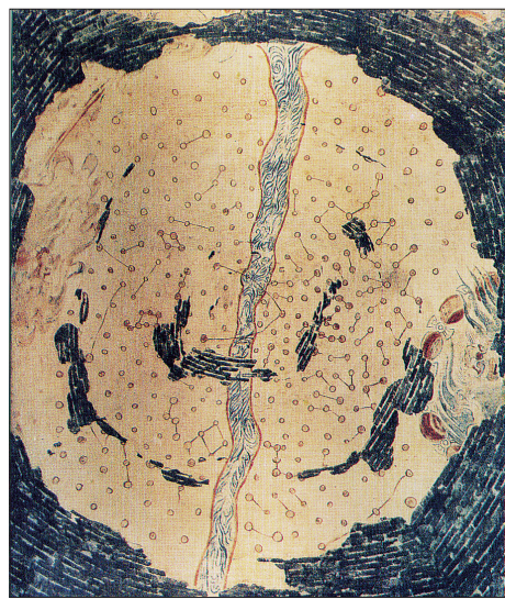
北魏元义墓中的天象图
