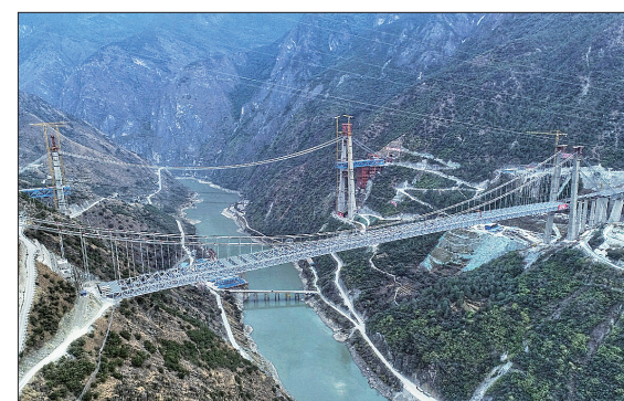
云南香丽高速公路虎跳峡金沙江特大桥合龙
