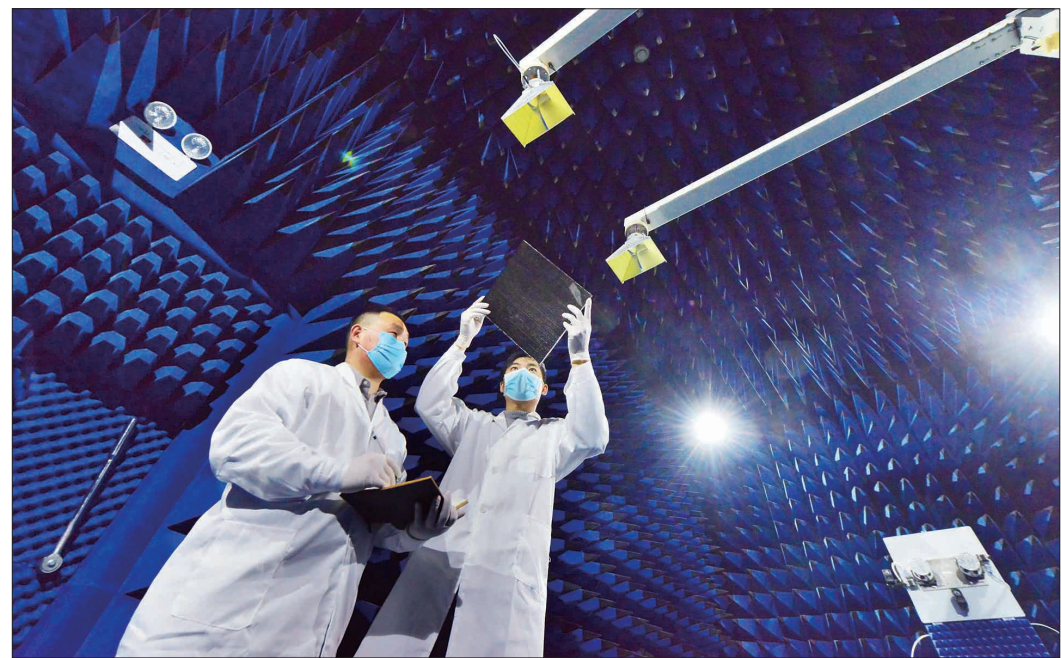
洛阳尖端技术研究院工作人员测试电磁吸波材料产品性能
