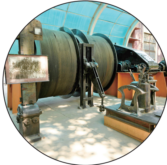
新中国首台直径2.5米双筒提升机
