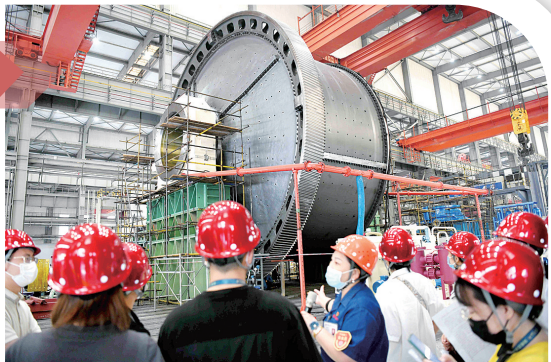
在中信重工了解超大型矿用磨机制造过程
