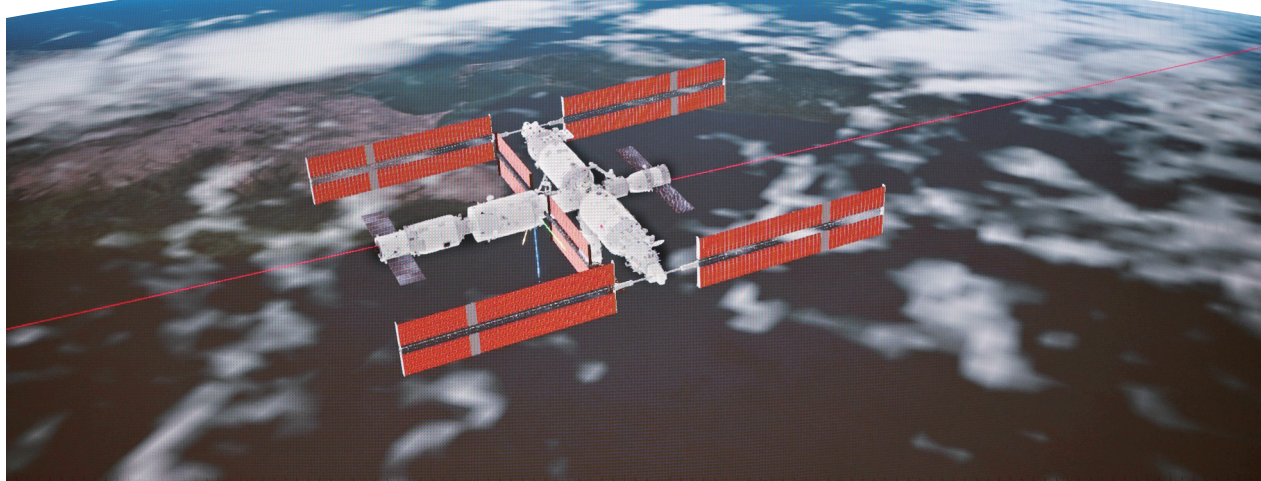
在北京航天飞行控制中心拍摄的成功对接后的神舟十八号载人飞船和空间站组合体的模拟画面 (新华社发)
